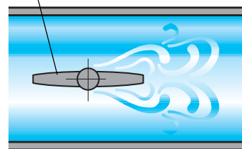
Turbulenzen bei Klappensteuerung
