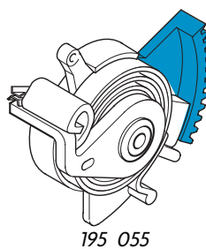
Zahnradsegment ohne GRA
