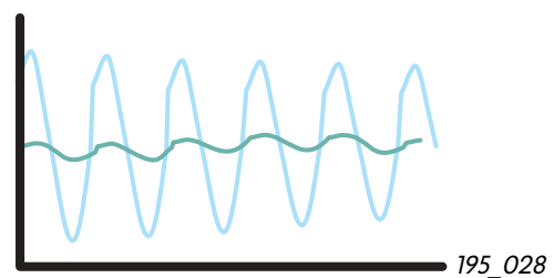
Schwingungsverhalten von Motor und Getriebe bei Leerlaufdrehzahl
